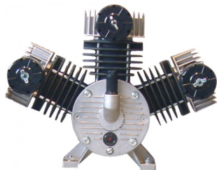
25387 Tête de compresseur 60CV3
